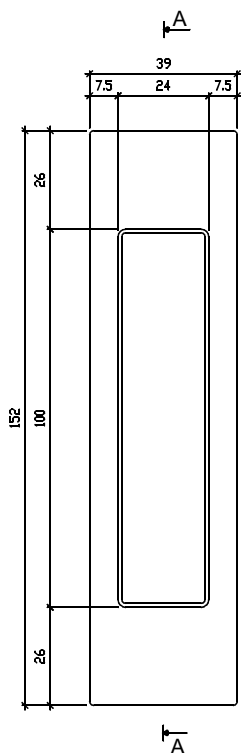
Widok z przodu uchwyt I
