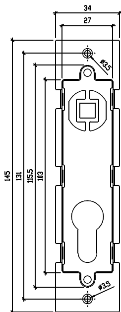
Widok z przodu rozeta montażowa II
