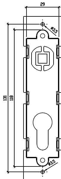
Widok z tyłu rozeta montażowa II
