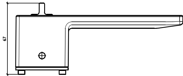
Widok z dołu klamka I (wariant z pokrętłem)
