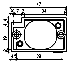
Widok z tyłu rozeta montażowa II
