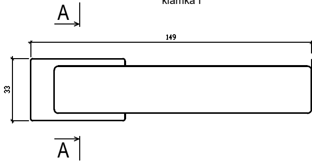
Widok z przodu klamka I
