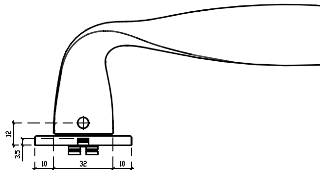
Widok z dołu klamka I
